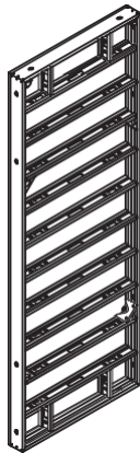
Елемент D 275 x 100 Стоманен елемент с 15 mm шперплат.
